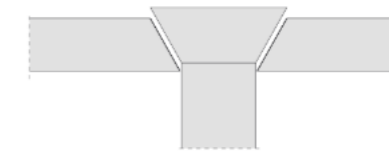
Przebicie stropu przez słup
